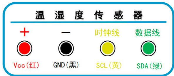
Vcc: 电源 (红色); GND (黑色); SCL (黄色或者白色); SDA (绿色或者蓝色)
