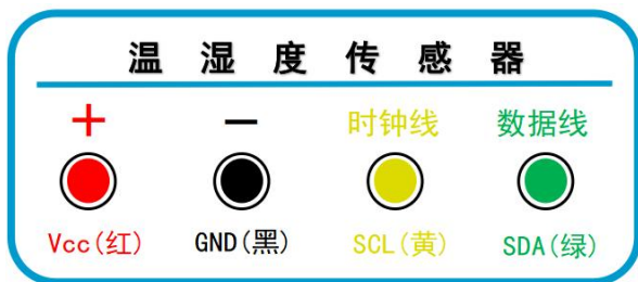
Vcc: 电源(红色); GND(黑色); SCL(黄色或者白色); SDA(绿色或者蓝色)
